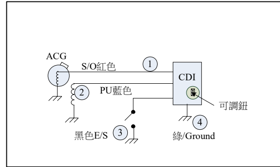
圖示四. 實車配線圖
